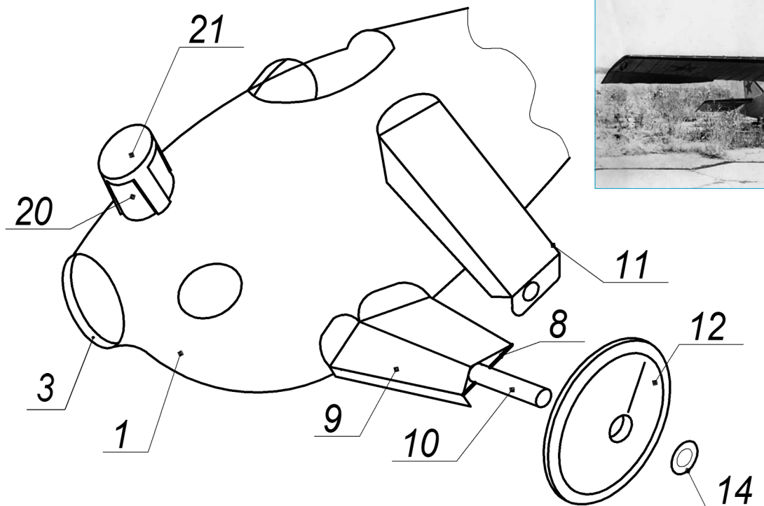
Рис. 5. Схема склейки шасси.
