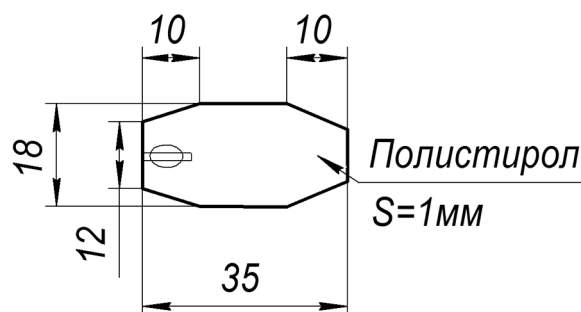
Рис. 5. Размеры лопасти весла.
