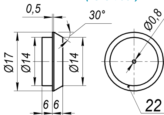
Рис. 3. Носовая бобышка (пенопласт).
